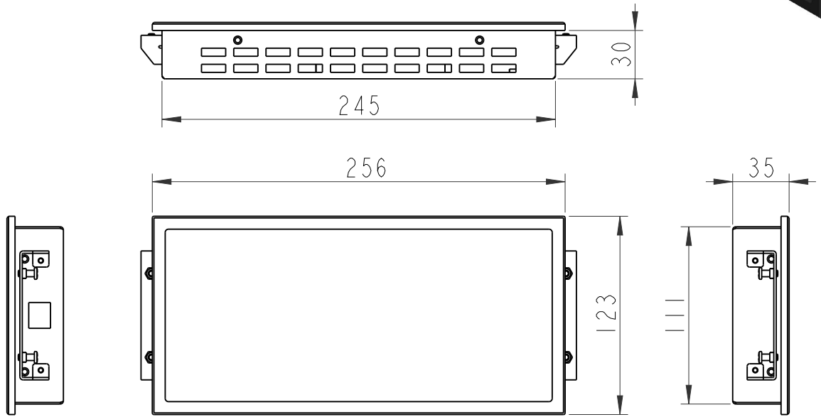
外形尺寸
